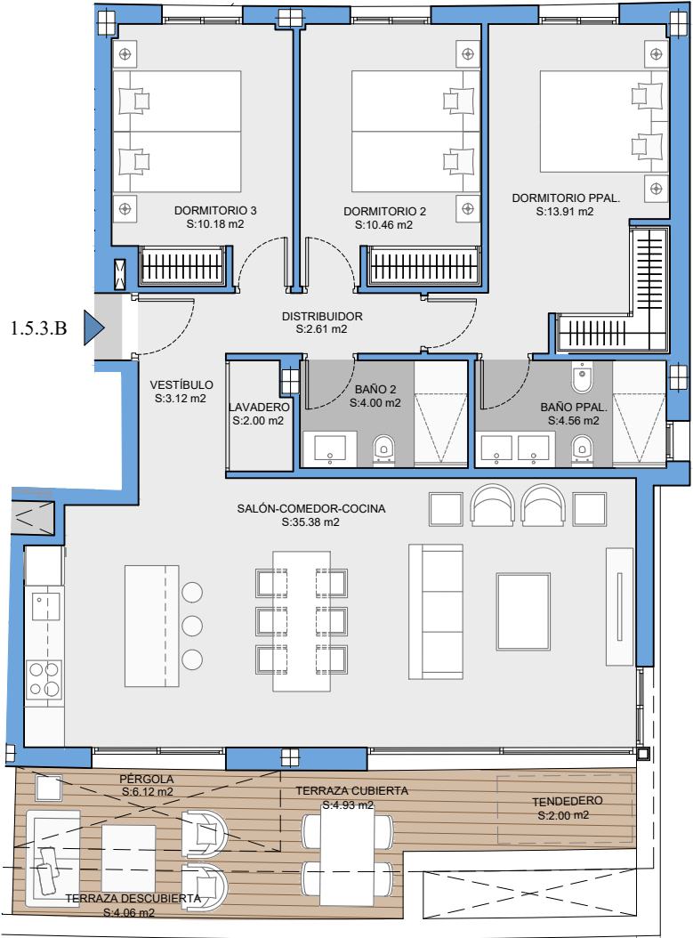
PLANTA SEGUNDA
